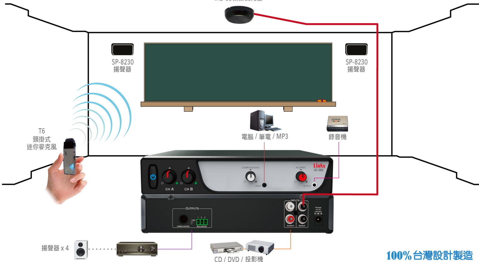
IRS-55頂掛受光器
